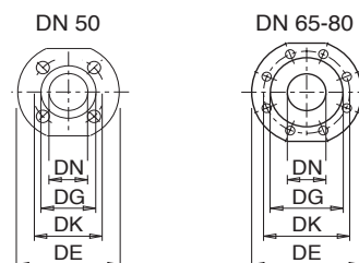
Flanges EN 1092-2 PN 25 - 40
